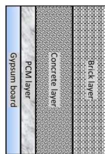
الف) دیوار شامل PCM
