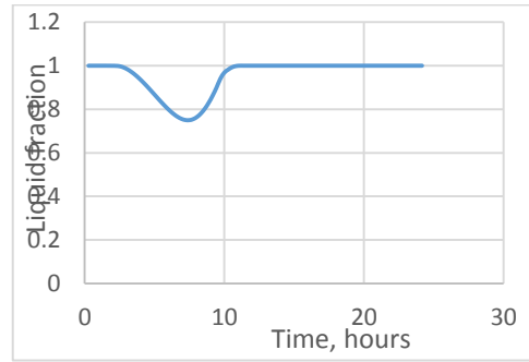
نمودار (۳-۴) - تغییرات جزء مایع مواد تغییر فاز دهنده بر حسب زمان
