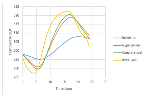
نمودار (۲-۳): تغییرات دمای میانگین هوای داخل ساختمان و دیوارها در حالتی که از pcm استفاده نشود
