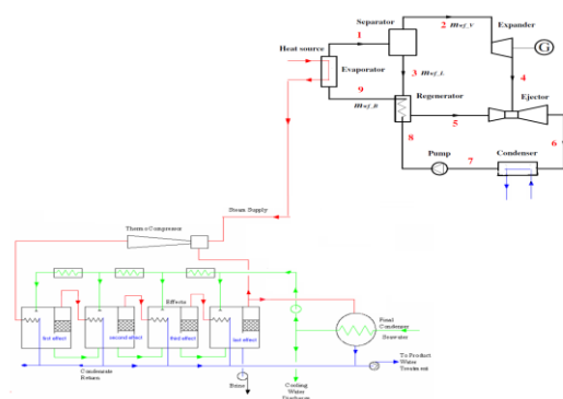
شکل (۶): دیاگرام کلی سیکل ترکیبی
