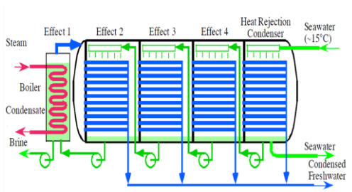
شکل (۳) : آب شیرین‌کن MED
