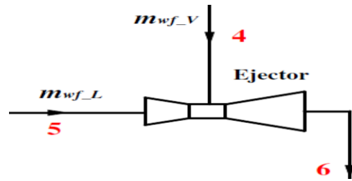
شکل (۱۰): اجکتور در سیکل کالینا
