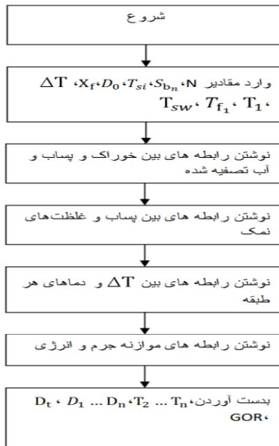
شکل (۱۴): فلوچارت تحلیل آب شیرین کن
