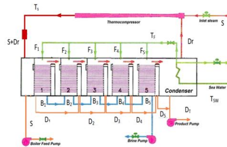
شکل (۱۲): نمودار جریان یک سیستم MED
