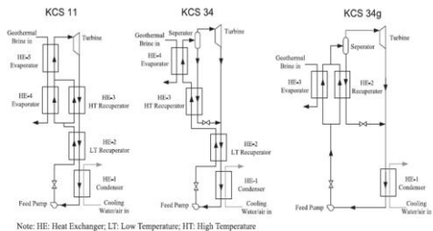
شکل (۲) : انواع سیکل کالینا
