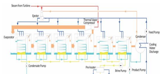
کل (۹): آب شیرین‌کن MED
