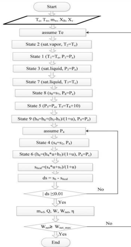
شکل (۱۳): فلوچارت تحلیل سیکل کالینا [۱۲]
