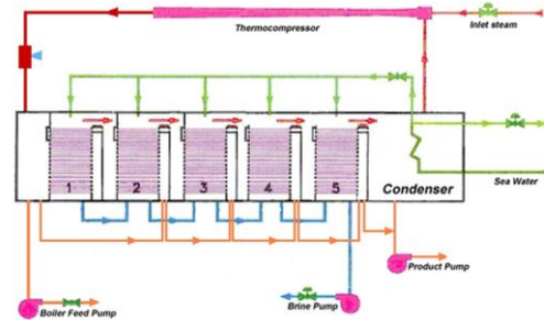
شکل (۴): آب شیرین کن MED-TVC
